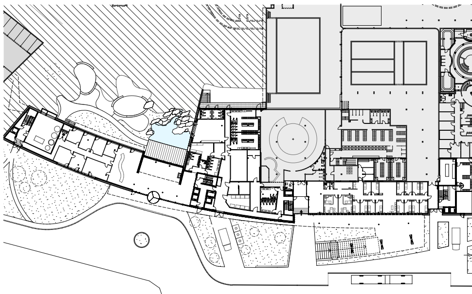
Plan général
